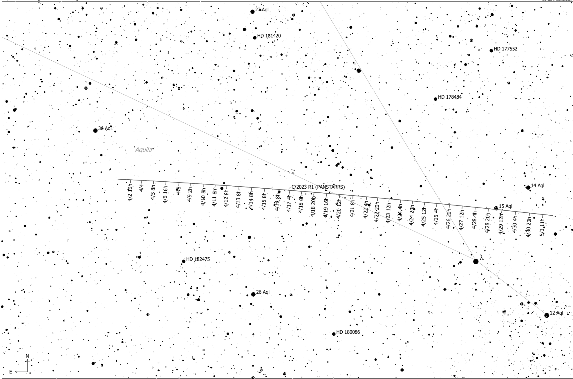
C/2023 R1 (PANSTARRS) (Comet)
